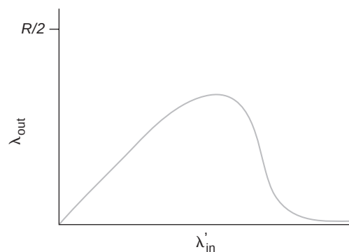
Figura 3.48 ♦ Escenario 3: rendimiento con buffers finitos y rutas con varios saltos.
