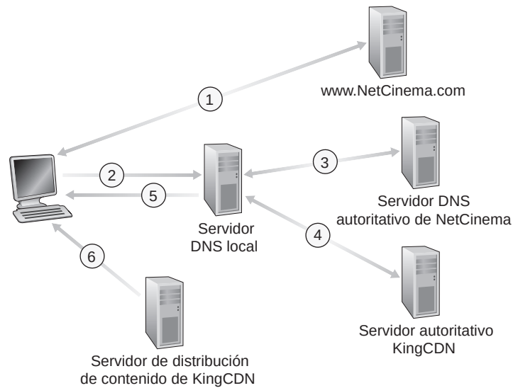
Figura 2.25 ♦ DNS redirige una solicitud de usuario hacia un servidor CDN.
