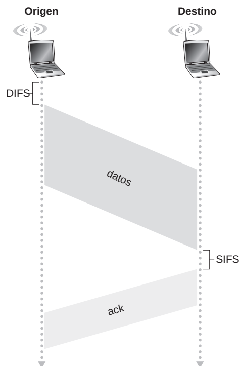
Figura 7.10 ♦ 802.11 utiliza reconocimientos (ACK) de la capa de enlace.
